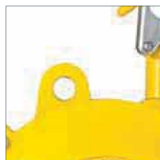
Öse für Sicherheitskette Nach DIN 15112 muss der Balancer mit einer zusätzlichen Sicherheitskette befestigt werden.
